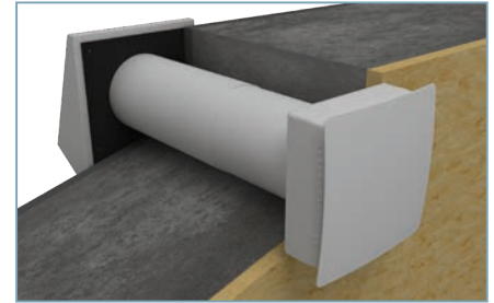
Montage in eine Standard- Wandstärke mit dem Einsatz der Außenhaube (Art. Nr. 50530)
