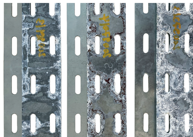
ZM - kontinuierliche Verzinkung mit Magnesium und Aluminiumbeimischung
